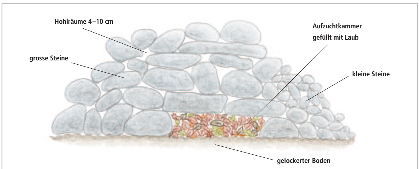
Abb. 15: Aufbau eines frisch gebauten Steinhäufens mit Aufzuchtchamber für Wiesel (falls für das Dach der Aufzuchtchamber keine genügend grossen Steine vorhanden sind, kann es auch mit Stammstücken gebaut werden).
